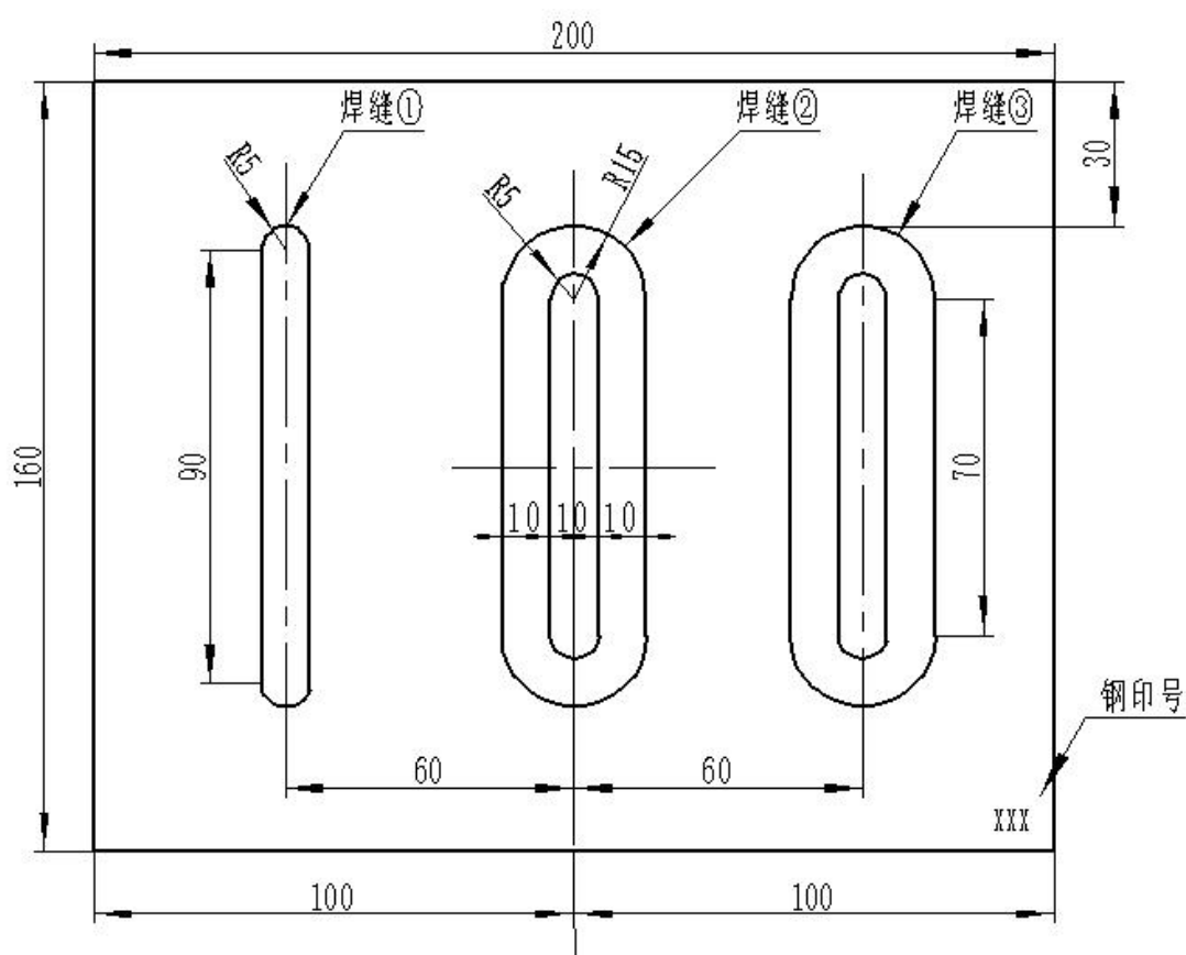
图 5：模块三焊接示意图
