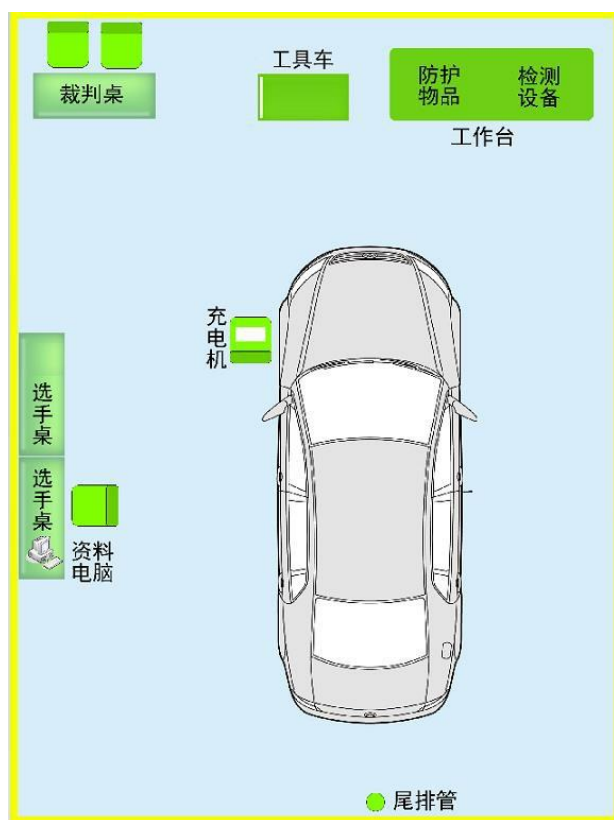
图 1 整车竞赛工位布置图
