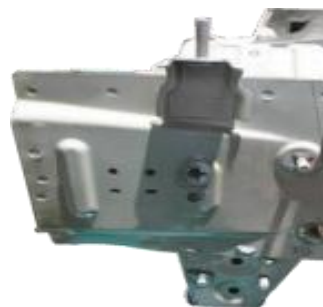
图4左前纵梁外侧
